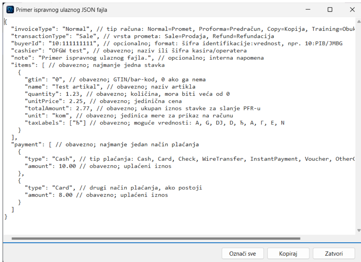
Slika 3: Primer ispravnog ulaznog JSON fajla.
